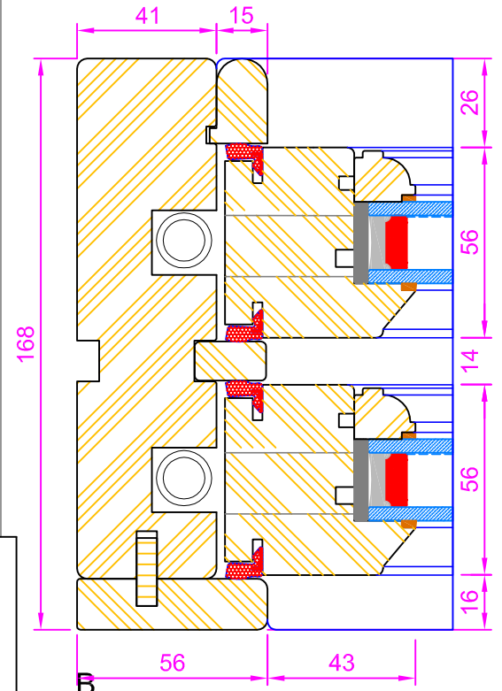
Section B-B (Dwg.No. 2006.1)
