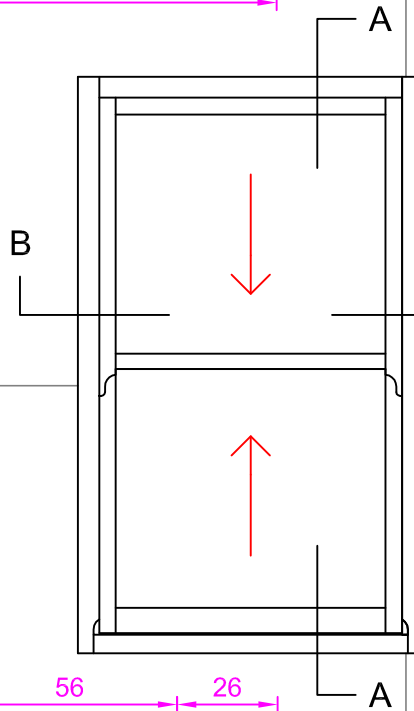
Section B-B (Dwg.No. 2006.1 mirr'd)
