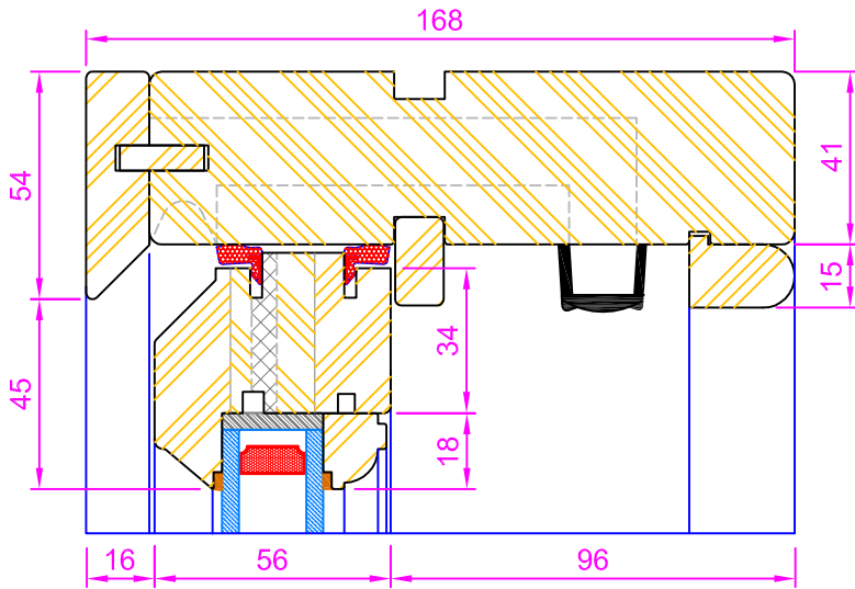
Section A-A (Dwg.No. 2003)
