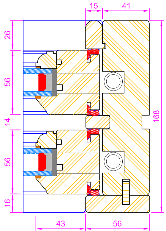
Section B-B (Dwg.No. 2006.1 mirr'd)
